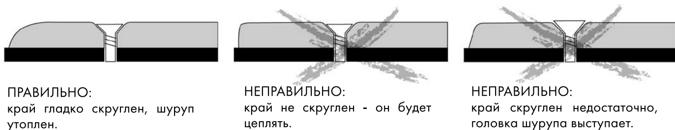
Рис. 5 Набойки - пластинки. Обработка краев.
